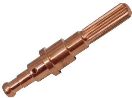
120036 ELETRODO DE CORTE 9 8215
